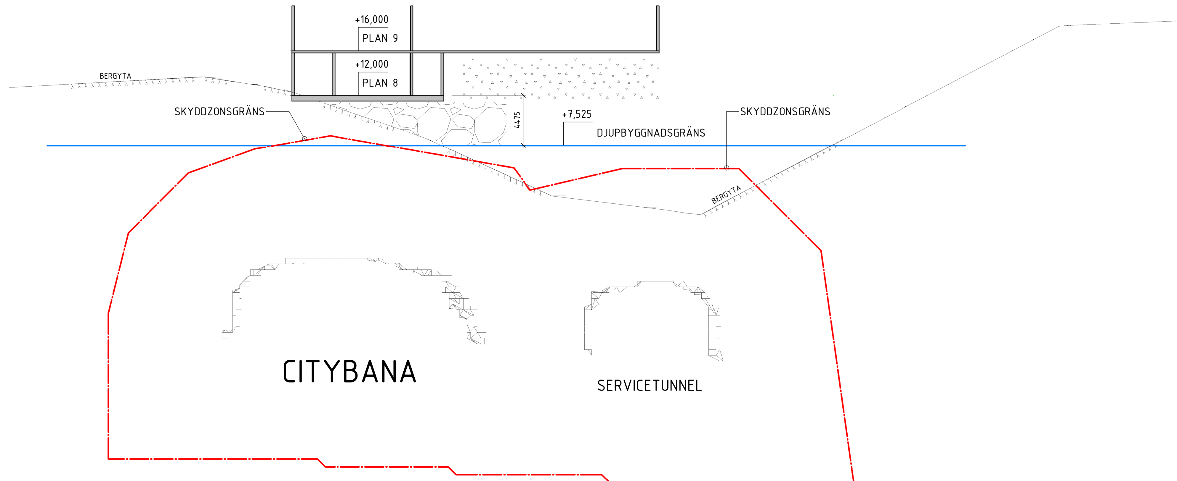
B-B 1 : 200
